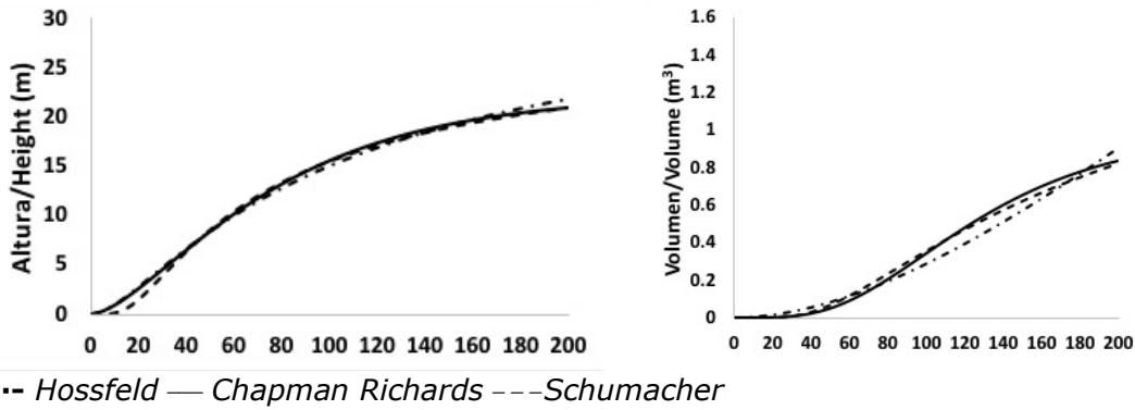
Figura 2. Tendencias del crecimiento promedio del diámetro normal, área basal, altura y volumen de los modelos de Chapman-Richards , Hossfeld I y Schumacher de Pinus leiophylla Schiede ex Schtdl. & Cham.
