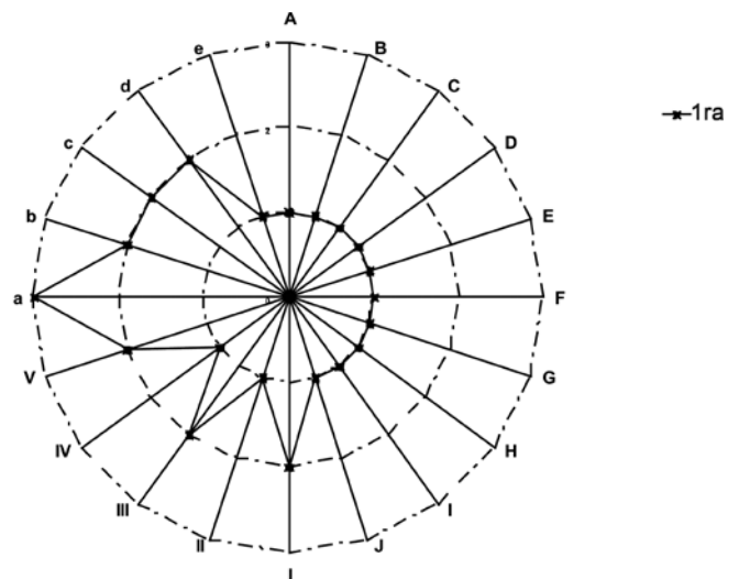
Criterio apilado: A = Uniformidad medida separador; B = Separador derecho uniforme; C = Alineación separadores; D = Distancia entre separadores; E = Ubicación final separador; F = Uniformidad travesaños; G = Alineación travesaños inferiores; H = Travesaños derechos; I = Apilado diferentes grosores; J = Apilado madera diferentes largos. Criterio operación de la estufa: I= Mantenimiento sistema inyección de calor; II= Calibración de velocidad de aire; III = Mantenimiento sistema humidificación; IV= Calibración sensores de temperatura; V= Calibración dispositivo control de humedad relativa. Criterio programa de secado: a = Ubicación de los sensores de humedad en tablas muestras; b = Seguimiento del programa de secado; c = Inspección de condiciones iniciales de la madera al iniciar proceso; d = Determinación del programa de secado; e = Determinación y aplicación de etapa acondicionamiento (enfriamiento). Stacking criterion: A = Uniform measures of dividers; B = Uniform straight dividers; C = Alignment of dividers; D = Distance between dividers; E = Final placing of dividers; F = Uniform crossbeams; G = Lower crossbeam alignment; H = Straight crossbeams; I = Stacking of different thicknesses; J = Stacking of lumber with different board lengths to be dried. Kiln operation criterion: I= Maintenance of the heat injection system; II= Air speed calibration; III = Maintenance of the moisturizing system; IV= Temperature sensor calibration; V= Calibration of the relative humidity control device. Drying program criterion: a = Location of the moisture sensors in the sample boards; b = Monitoring of the drying program; c = Inspection of the state of lumber at the beginning of the process; d = Definition of the drying program; e = Determination and application of the conditioning (cooling) stage.
