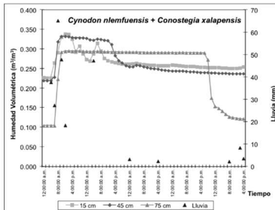
Figura 2. Comportamiento de la humedad del suelo en cinco usos del suelo localizados en una zona de recarga durante el impacto del durante el huracán Dean (22 de agosto 2007).
