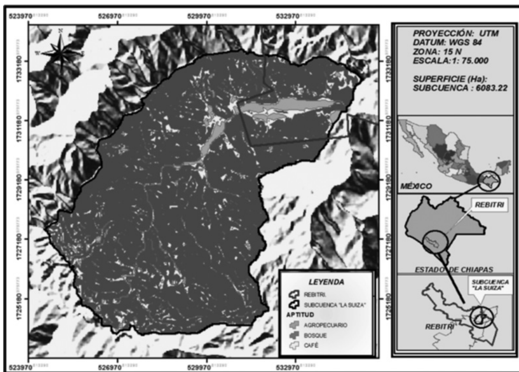
Figura 4. Aptitud del uso suelo en la microcuenca La Suiza, Chiapas. Figure 4. Land use ability in La Suiza watershed, Chiapas .
